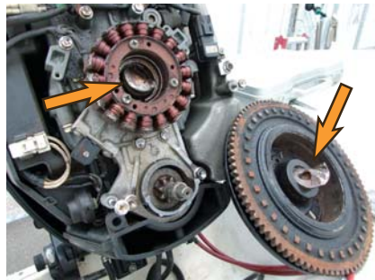
折れたクランクシャフト
